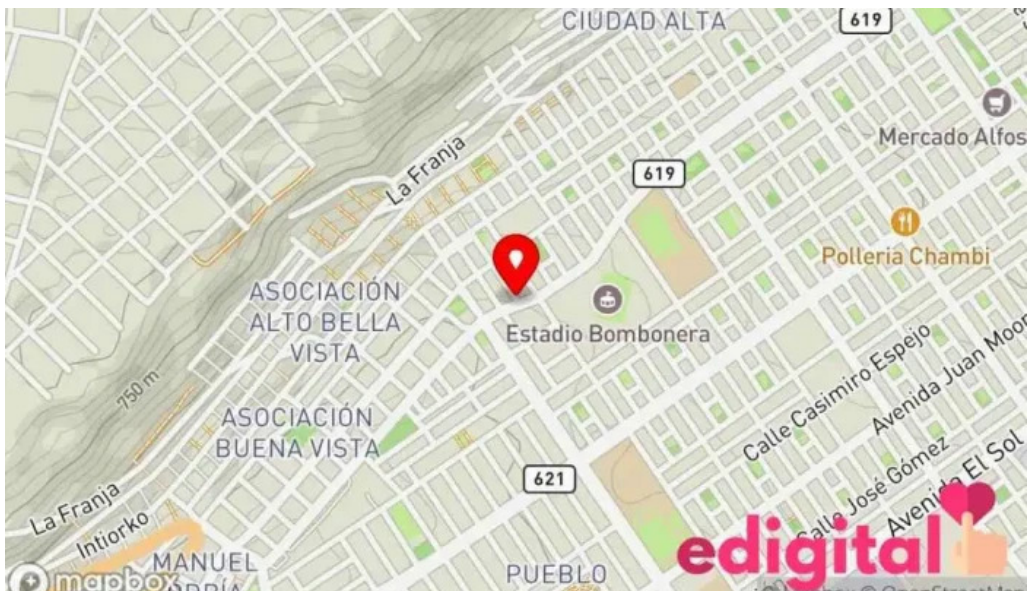
Farmacia mapa
